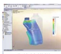
非线性模拟
